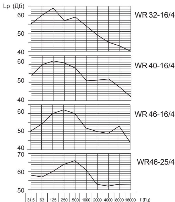
Уровень шума
