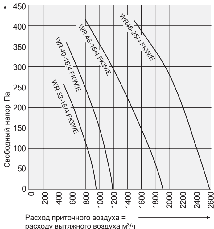
Расход воздуха
